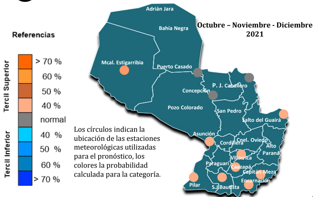
Figura 5. Pronóstico de Temperatura media trimestre OND 2021.
