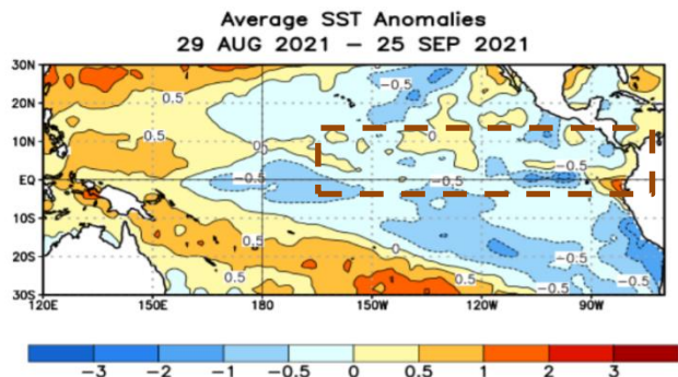
Figura 1. Anomalía de la temperatura superficial del mar en °C promediada en la semana del 29 de agosto al 25 de setiembre de 2021. Fuente: IRI. (Instituto Internacional de Investigación para el Clima y la Sociedad).
