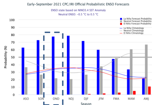
Figura 2. Probabilidad de fases del ENSO para la región de El Niño 3.4 actualizado al 09 de setiembre de 2021. Fuente: IRI (Instituto Internacional de Investigación para el Clima y la Sociedad).
