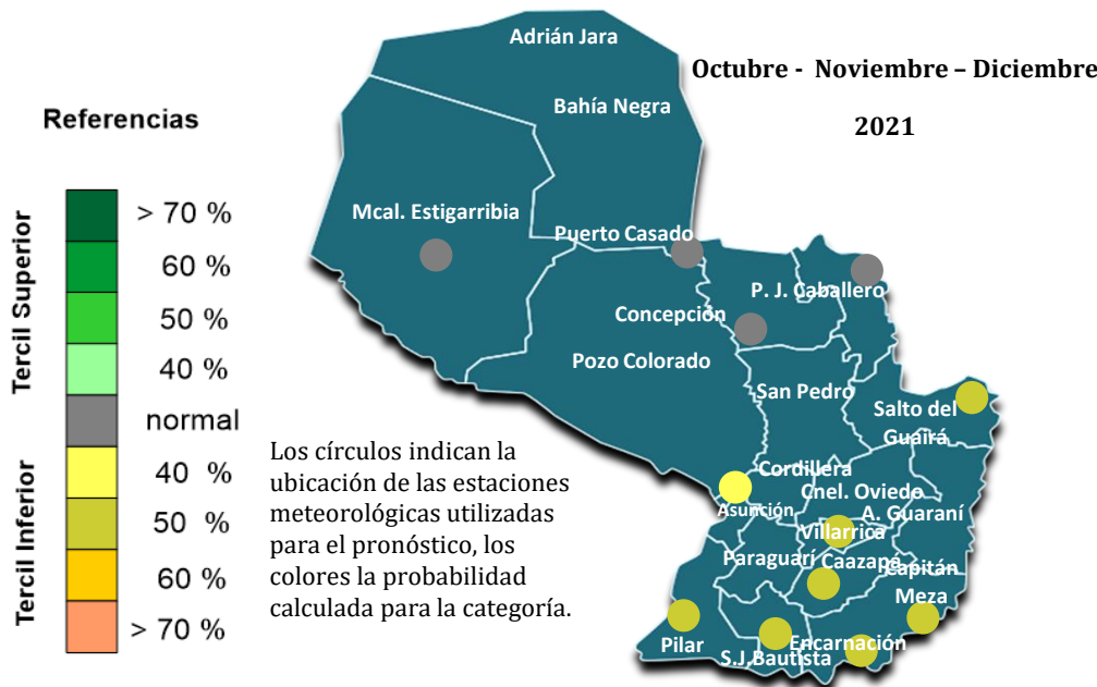
Figura 4. Pronóstico de Precipitación trimestre OND 2021.
