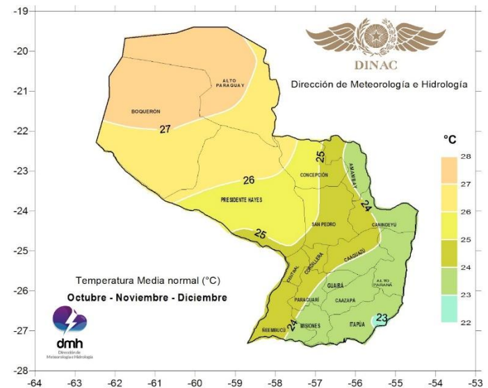
Figura 9. Temperatura media normal. OND.
