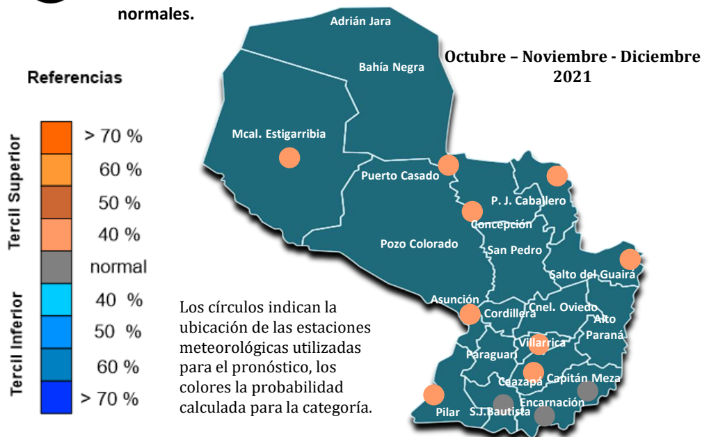
Figura 7. Pronóstico de temperatura mínima media. OND 2021.
